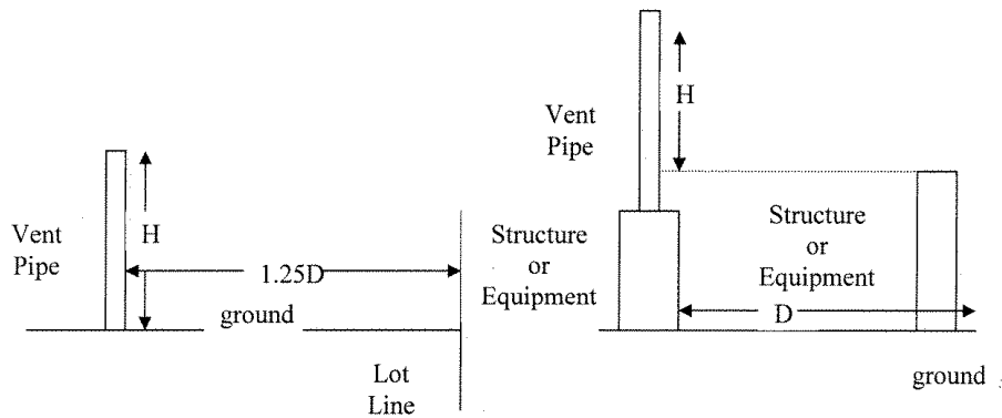
Figure 2209.5.4.3.4 Hydrogen vent pipe height (H) versus distance (D) requirements
